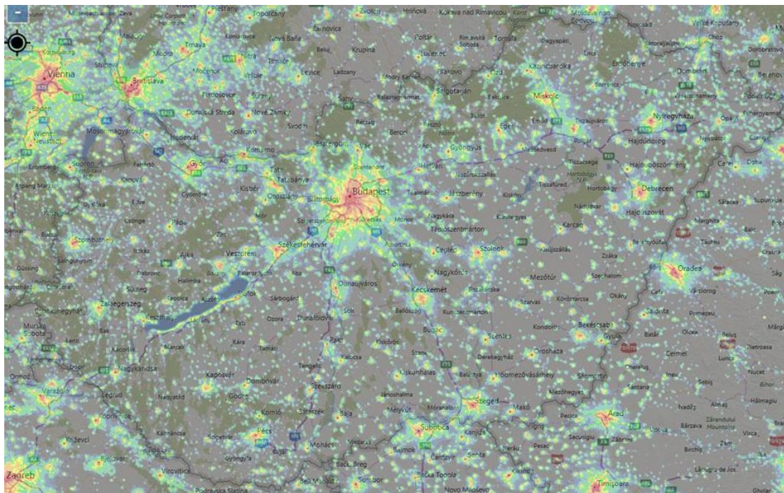
13. ábra: Magyarország indikatív fényterhelése (Műholdfotó, 2015.)
